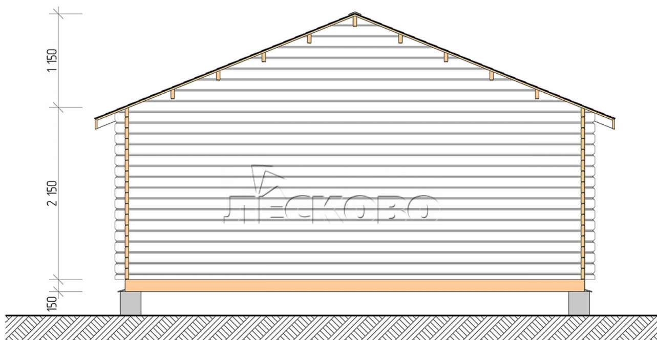
Разрез
